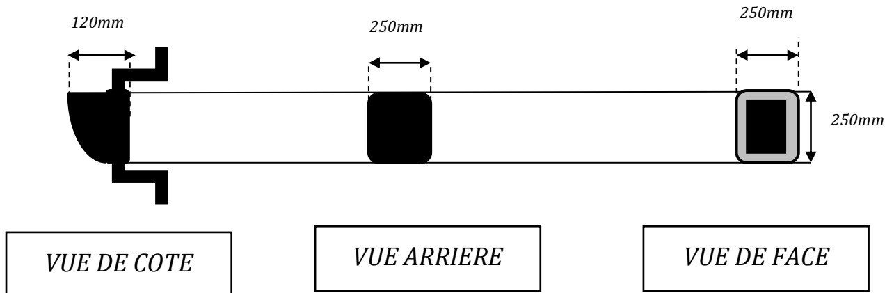
Dimension de la lanterne
