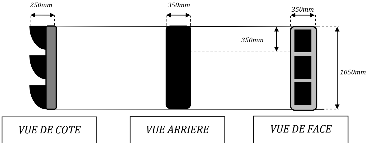
Dimension de la lanterne
