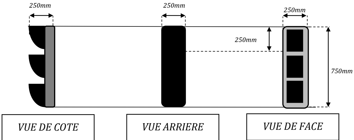
Dimension de la lanterne
